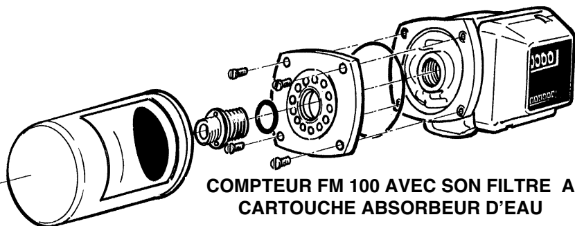
GROUPES DE POMPAGE M240 ÉQUIPÉ D'UN COMPTEUR MÉCANIQUE FM
